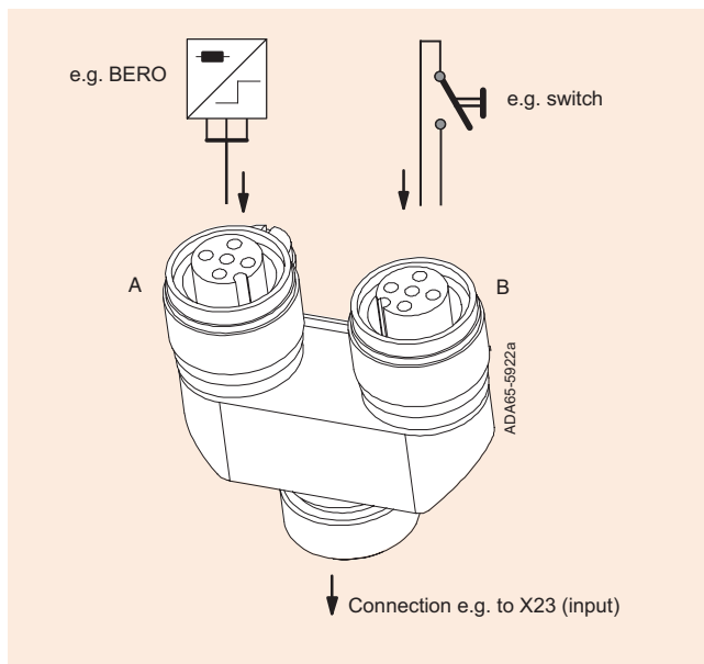
Y connector
