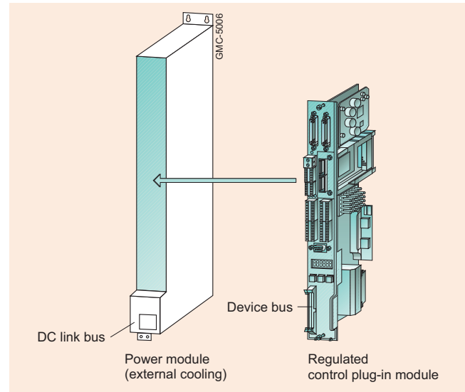
Drive module
